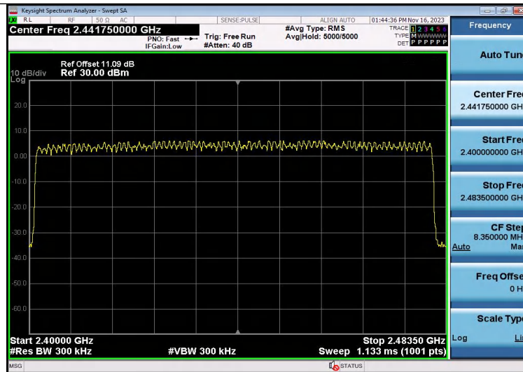
\pi/4 DQPSK Modulation
