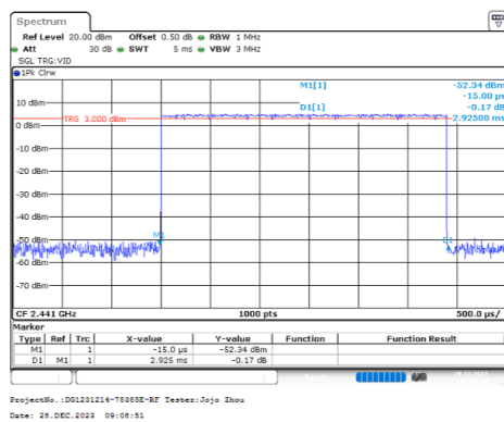
PI/4-DQPSK_Hopping_2DH5
