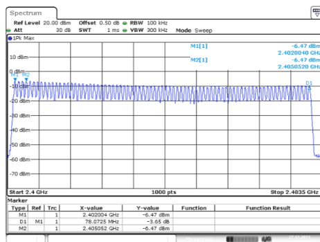
GFSK_Hopping_DH1
