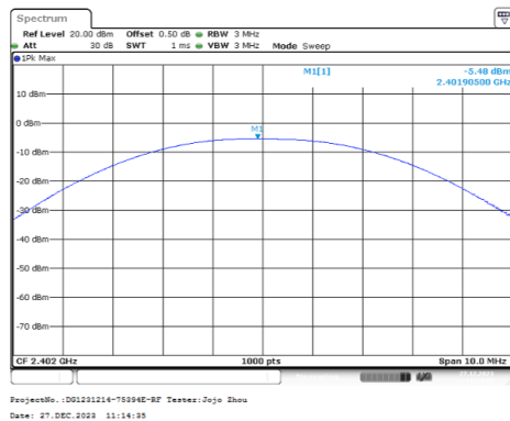
GFSK_Low_DH1
