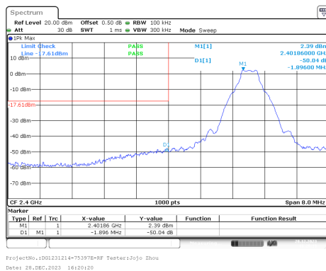
GFSK_Low_DH1
