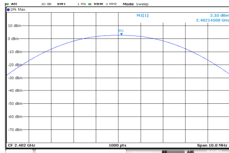
GFSK_Low_DH1
