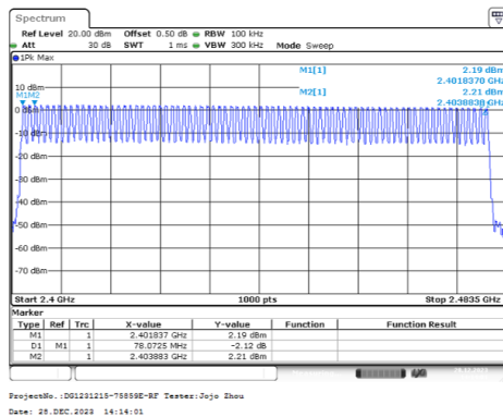
GFSK_Hopping_DH1
