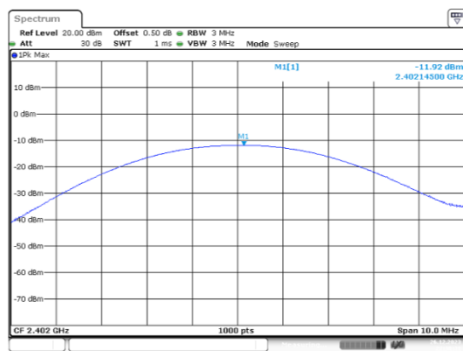
GFSK_Low_DH1
