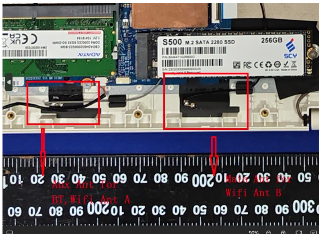
2) EUT Photo
