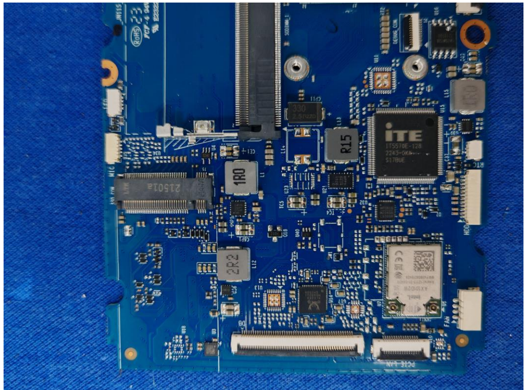
18) EUT Photo
