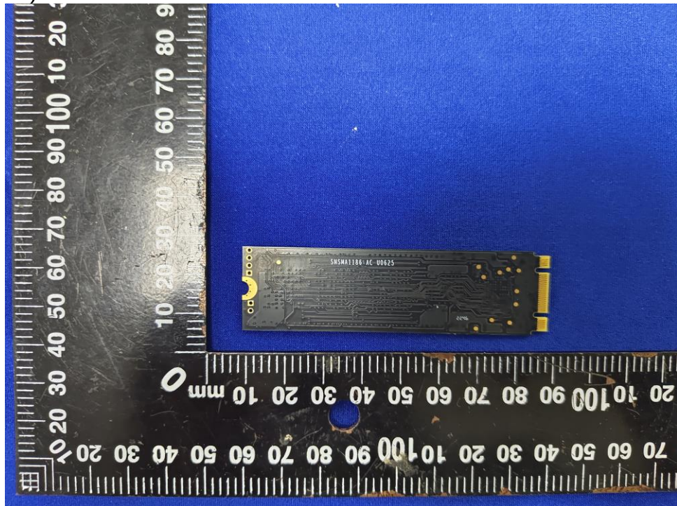
11) EUT Photo
