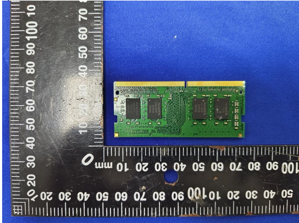
10) EUT Photo
