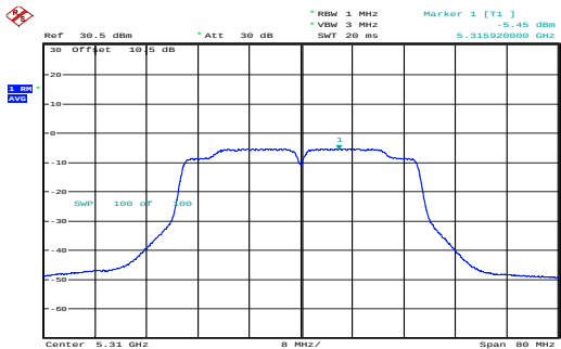
n40_5310MHz_Chain 0 -5.45dBm/MHz
