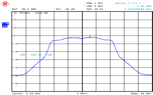
n20_5260MHz_Chain 0 -2.38dBm/MHz
