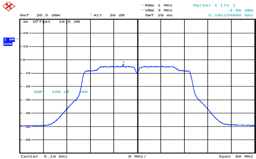
n40_5190MHz_Chain 0 -4.88dBm/MHz
