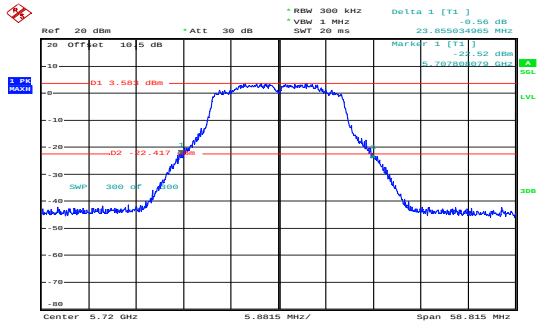
a_5720MHz_Chain 0 23.855MHz
