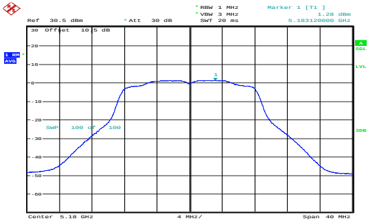
a_5180MHz_Chain 0 1.28dBm/MHz
