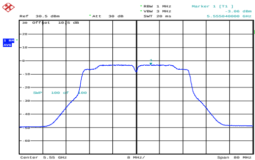
n40_5550MHz_Chain 1 -3.06dBm/MHz
