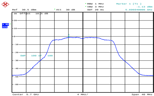
n20_5700MHz_Chain 0 -1.13dBm/MHz
