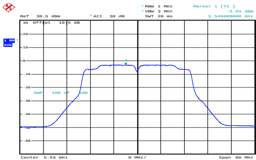
n40_5550MHz_Chain 0 -3.04dBm/MHz
