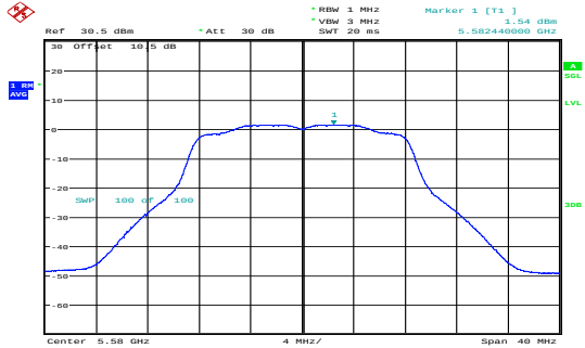
a_5580MHz_Chain 1 1.54dBm/MHz
