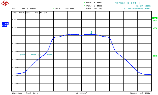
a_5200MHz_Chain 0 1.24dBm/MHz
