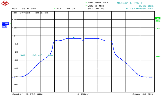
a_5785MHz_Chain 0 -3.05dBm/MHz
