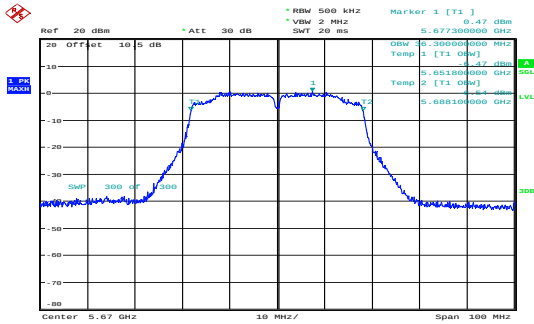
n40_5670MHz_Chain 0 36.300MHz
