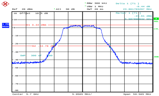
a_5700MHz_Chain 0 23.862MHz
