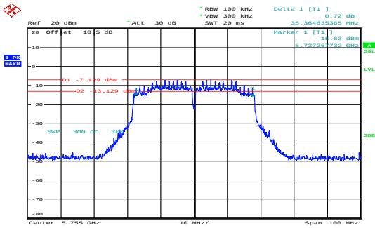
n40_5755MHz_Chain 0 35.365MHz
