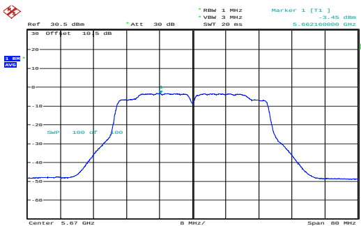
n40_5670MHz_Chain 1 -3.45dBm/MHz
