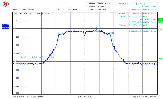
n40_5795MHz_Chain 0 36.300MHz
