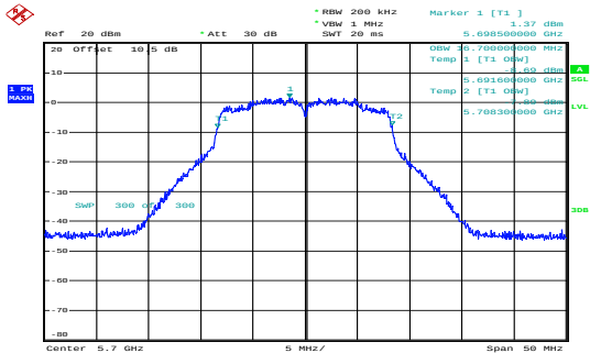
a_5700MHz_Chain 0 16.700MHz
