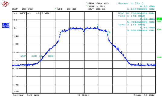
a_5500MHz_Chain 0 16.700MHz
