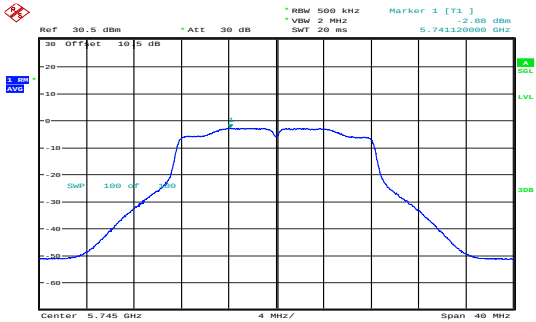
a_5745MHz_Chain 0 -2.88dBm/MHz
