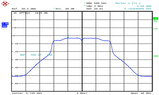
a_5745MHz_Chain 1 -3.06dBm/MHz
