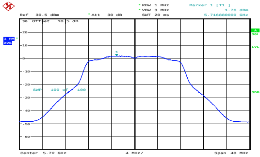
a_5720MHz_Chain 0 1.76dBm/MHz
