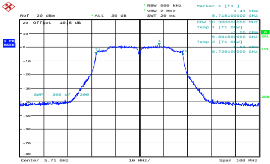
n40_5710MHz_Chain 0 36.300MHz
