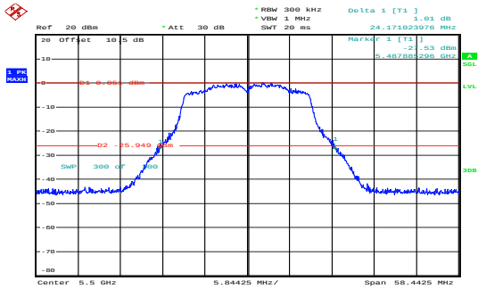
n20_5500MHz_Chain 0 24.171MHz
