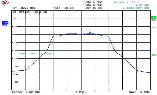
a_5320MHz_Chain 0 1.34dBm/MHz
