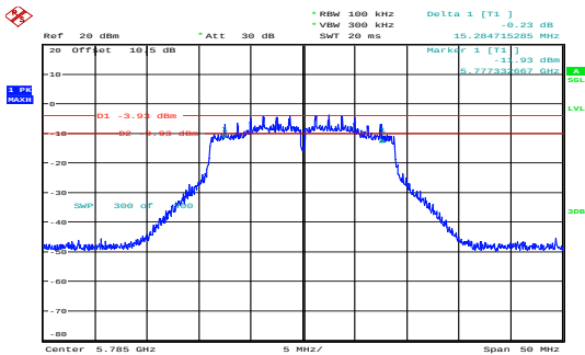
n20_5785MHz_Chain 0 15.285MHz
