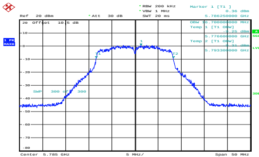
a_5785MHz_Chain 0 16.700MHz
