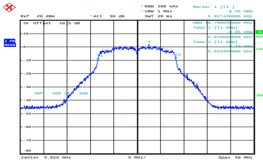
a_5825MHz_Chain 0 16.700MHz
