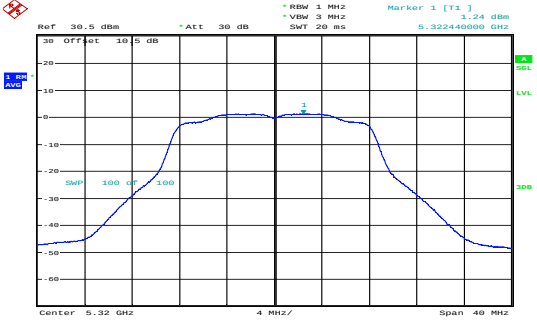
a_5320MHz_Chain 1 1.24dBm/MHz
