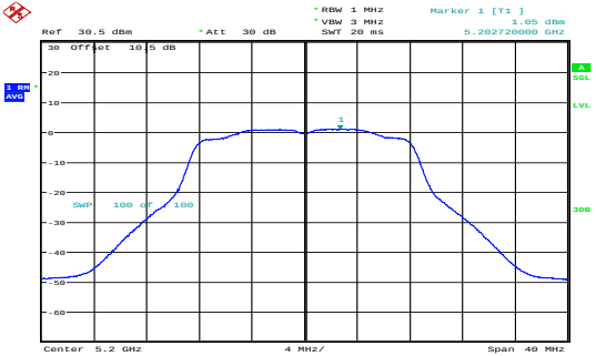
a_5200MHz_Chain 1 1.05dBm/MHz
