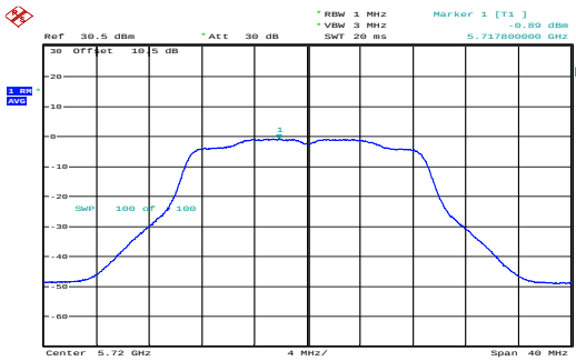
n20_5720MHz_Chain 1 -0.89dBm/MHz
