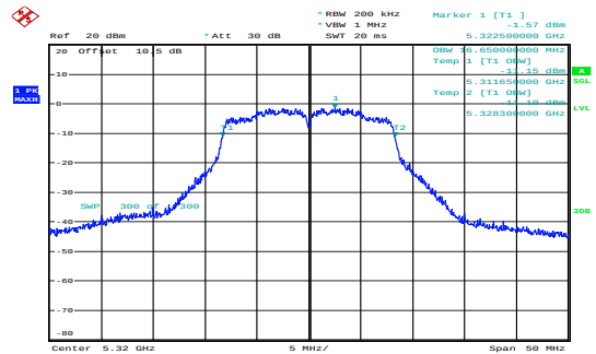
a_5320MHz_Chain 0 16.650MHz
