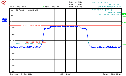
ac80_5210MHz_Chain 0 82.517MHz
