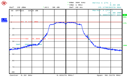
a_5320MHz_Chain 0 23.180MHz
