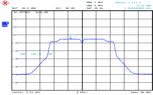
n40_5510MHz_Chain 0 -5.15dBm/MHz
