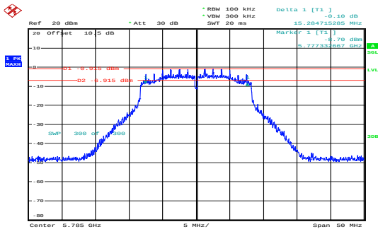
a_5785MHz_Chain 0 15.285MHz
