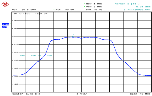
n20_5720MHz_Chain 0 -0.91dBm/MHz
