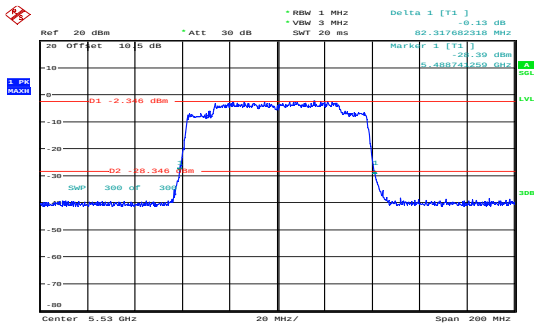
ac80_5530MHz_Chain 0 82.318MHz
