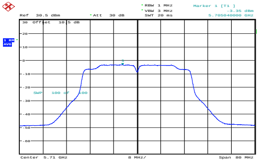
n40_5710MHz_Chain 1 -3.35dBm/MHz
