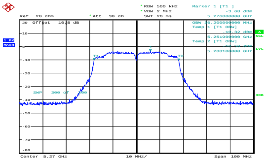
n40_5270MHz_Chain 0 36.200MHz
