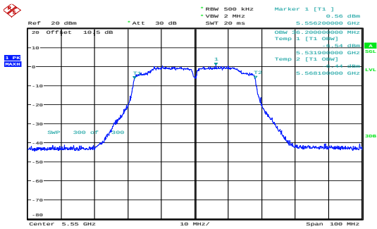
n40_5550MHz_Chain 0 36.200MHz
