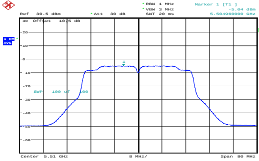
n40_5510MHz_Chain 1 -5.04dBm/MHz
