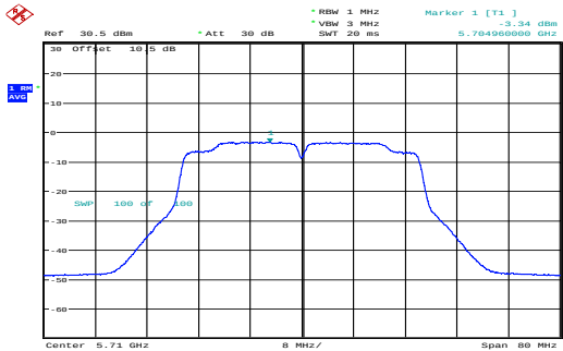
n40_5710MHz_Chain 0 -3.34dBm/MHz
