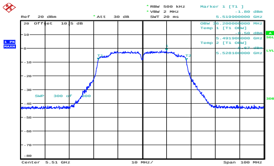
n40_5510MHz_Chain 0 36.200MHz
