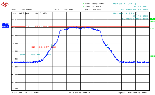
n20_5720MHz_Chain 0 23.747MHz
