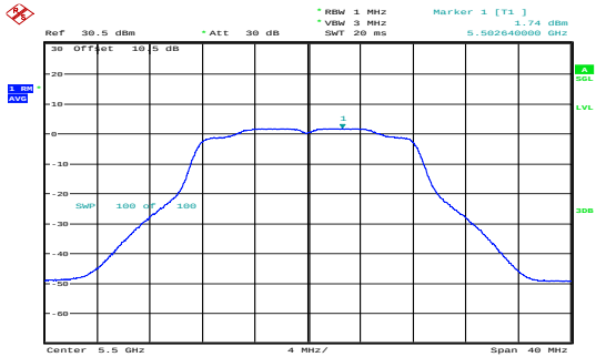
a_5500MHz_Chain 0 1.74dBm/MHz
