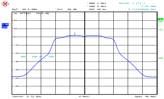
a_5720MHz_Chain 1 1.63dBm/MHz
