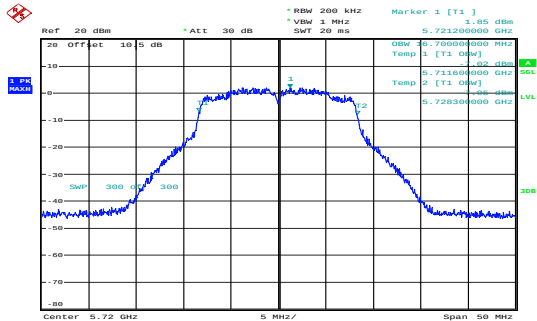
a_5720MHz_Chain 0 16.700MHz
