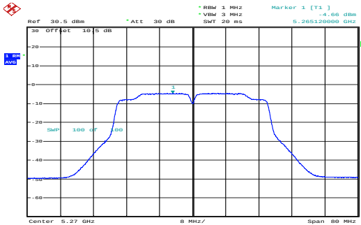
n40_5270MHz_Chain 1 -4.66dBm/MHz
