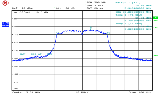
n40_5310MHz_Chain 0 36.300MHz
