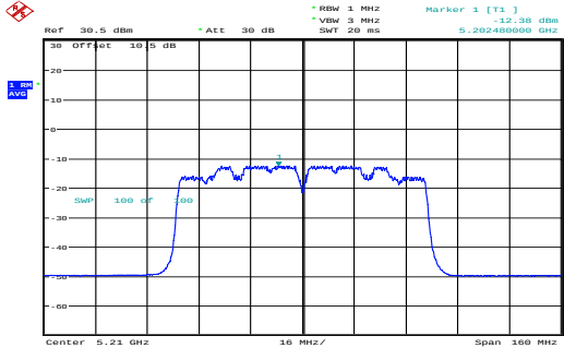
ac80_5210MHz_Chain 0 -12.38dBm/MHz
