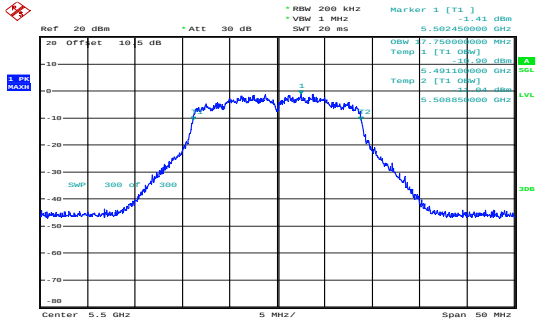
n20_5500MHz_Chain 0 17.750MHz
