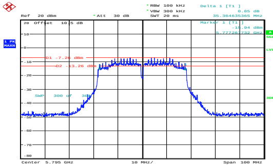
n40_5795MHz_Chain 0 35.365MHz
