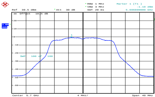
n20_5700MHz_Chain 1 -1.10dBm/MHz
