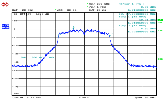
n20_5720MHz_Chain 0 17.750MHz
