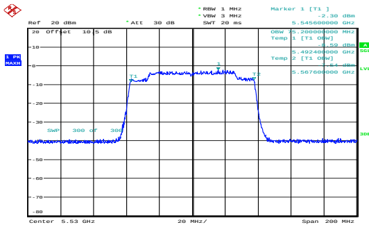
ac80_5530MHz_Chain 0 75.200MHz
