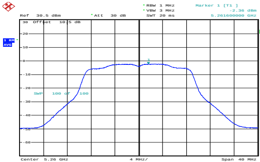
n20_5260MHz_Chain 1 -2.36dBm/MHz
