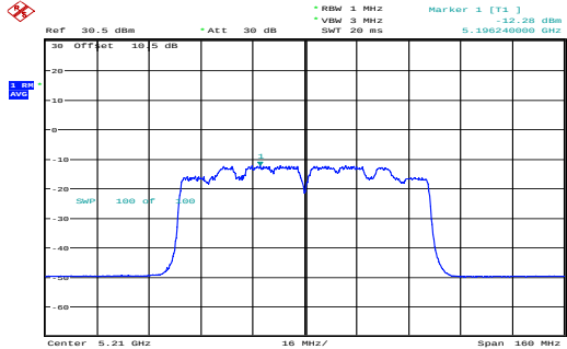
ac80_5210MHz_Chain 1 -12.28dBm/MHz
