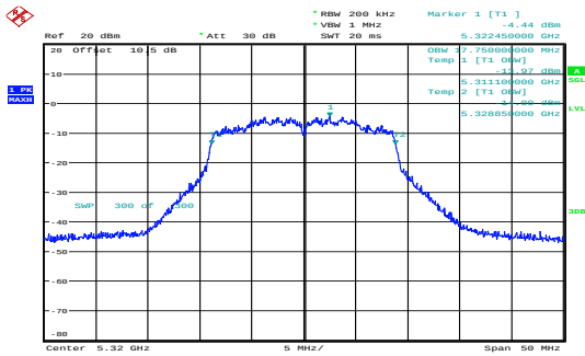
n20_5320MHz_Chain 0 17.750MHz
