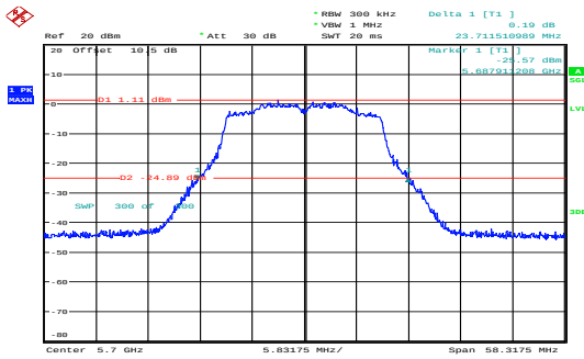
n20_5700MHz_Chain 0 23.712MHz
