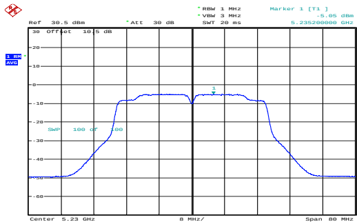
n40_5230MHz_Chain 1 -5.05dBm/MHz
