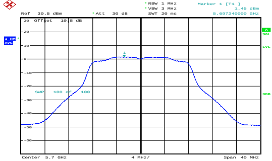
a_5700MHz_Chain 1 1.45dBm/MHz
