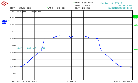
n20_5825MHz_Chain 1 -6.36dBm/MHz
