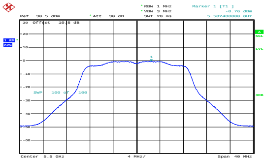
n20_5500MHz_Chain 0 -0.76dBm/MHz
