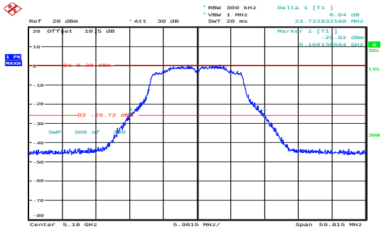
a_5180MHz_Chain 0 23.723MHz
