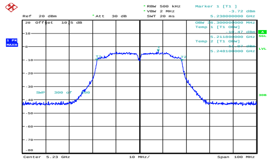
n40_5230MHz_Chain 0 36.300MHz
