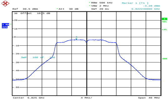
a_5825MHz_Chain 1 -3.28dBm/MHz
