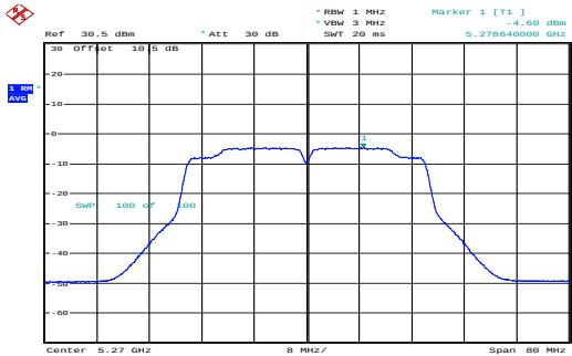
n40_5270MHz_Chain 0 -4.60dBm/MHz
