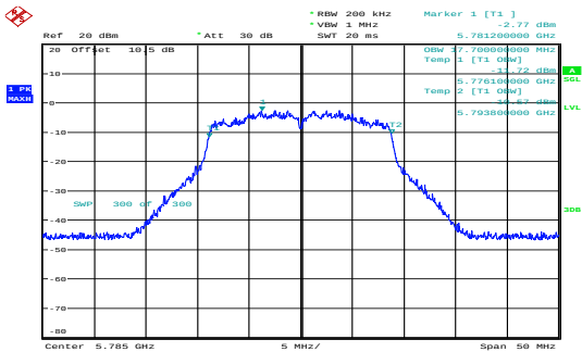
n20_5785MHz_Chain 0 17.700MHz
