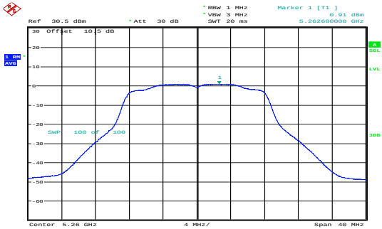
a_5260MHz_Chain 0 0.91dBm/MHz
