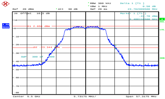
a_5500MHz_Chain 0 23.763MHz
