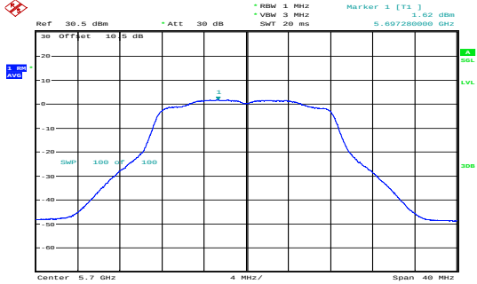
a_5700MHz_Chain 0 1.62dBm/MHz
