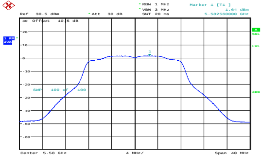
a_5580MHz_Chain 0 1.64dBm/MHz
