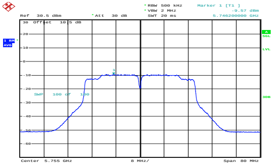
n40_5755MHz_Chain 1 -9.57dBm/MHz
