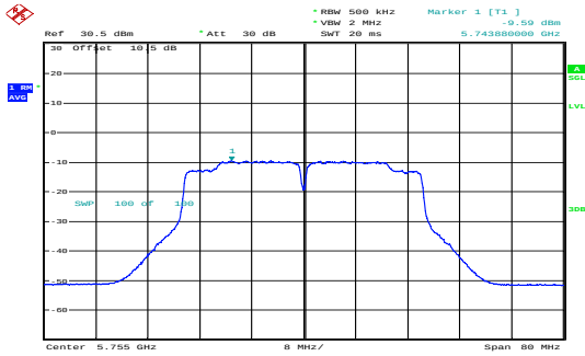
n40_5755MHz_Chain 0 -9.59dBm/MHz
