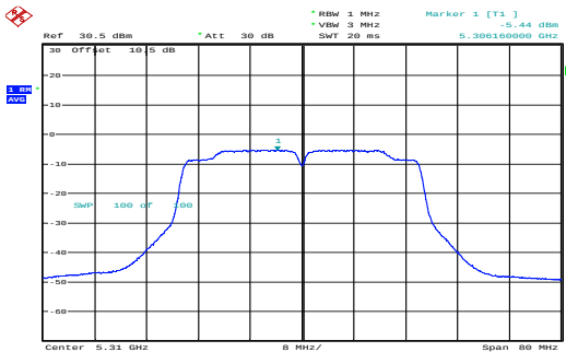
n40_5310MHz_Chain 1 -5.44dBm/MHz
