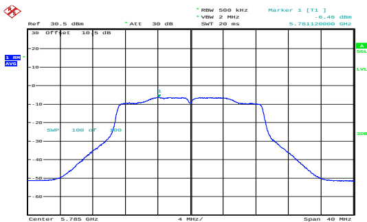
n20_5785MHz_Chain 0 -6.46dBm/MHz
