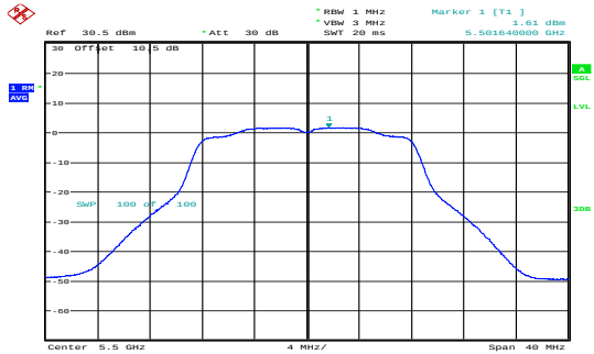
a_5500MHz_Chain 1 1.61dBm/MHz
