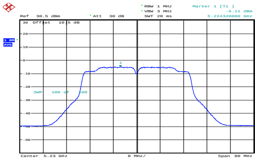
n40_5230MHz_Chain 0 -5.11dBm/MHz
