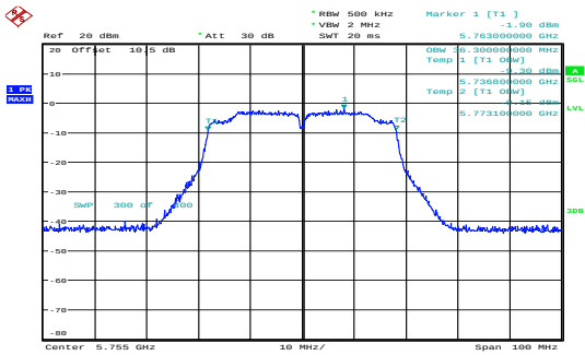
n40_5755MHz_Chain 0 36.300MHz
