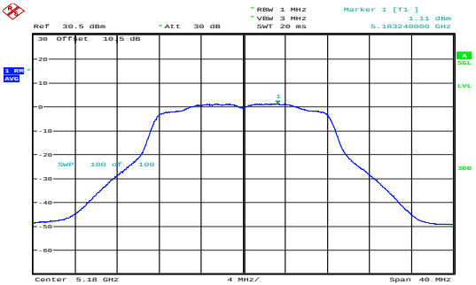
a_5180MHz_Chain 1 1.11dBm/MHz
