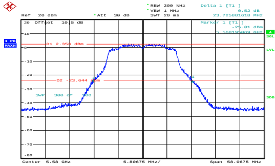
a_5580MHz_Chain 0 23.726MHz
