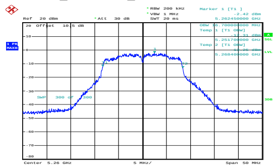
a_5260MHz_Chain 0 16.700MHz
