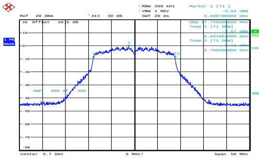
n20_5700MHz_Chain 0 17.750MHz
