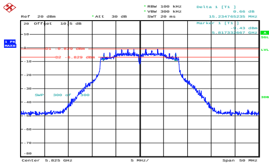
a_5825MHz_Chain 0 15.235MHz
