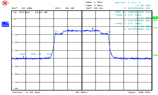
ac80_5290MHz_Chain 0 75.200MHz
