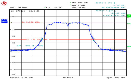
n40_5710MHz_Chain 0 44.855MHz
