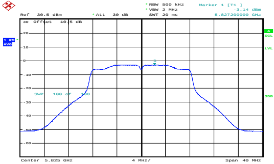
a_5825MHz_Chain 0 -3.14dBm/MHz
