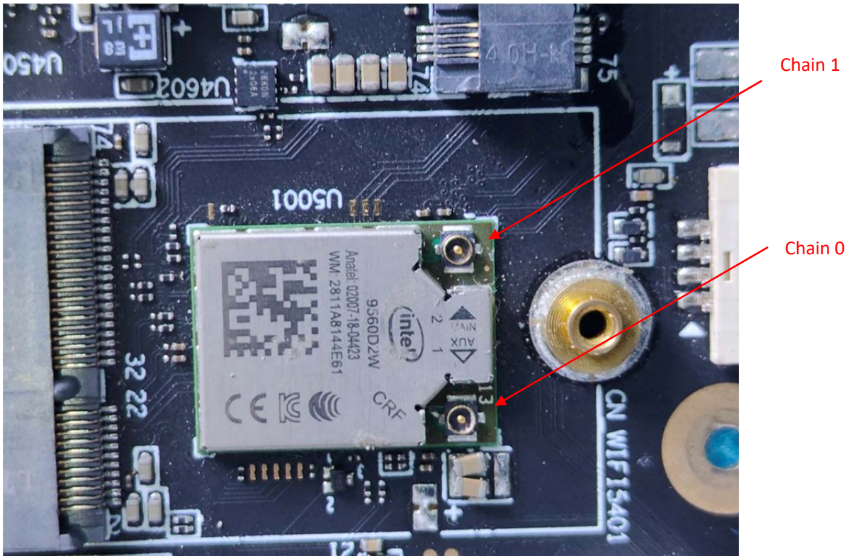
RF Module
