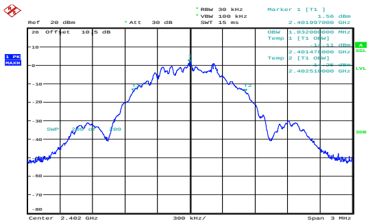
Low 1.032MHz
