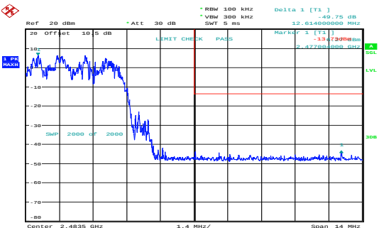
8DPSK_Hopping_Upper 49.75dB
