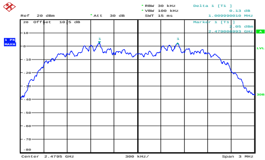
\pi/4 -DQPSK_High 1.010MHz
