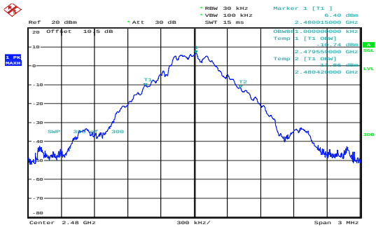
GFSK_High 0.861MHz
