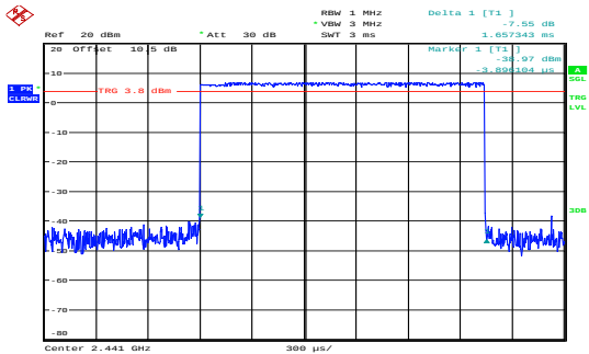
\pi/4 -DQPSK_Hopping_2DH3 1.657ms
