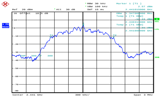
\pi/4 -DQPSK_Middle 1.347MHz
