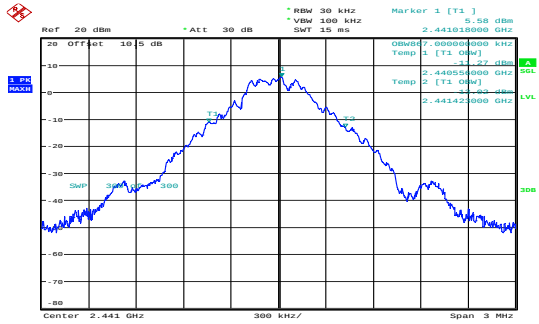
GFSK_Middle 0.867MHz
