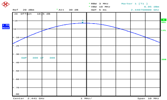
\pi/4 -DQPSK_Middle 6.95dBm
