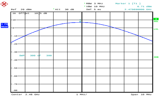
\pi/4 -DQPSK_High 6.71dBm
