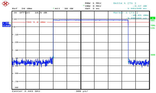
GFSK_Hopping_DH3 1.651ms
