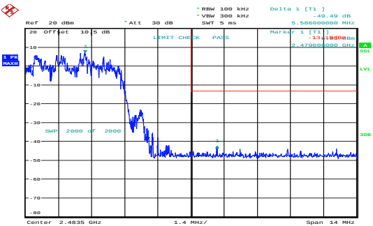
\pi/4 -DQPSK_Hopping_Upper 49.49dB
