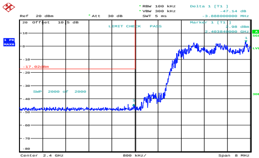
\pi/4 -DQPSK_Hopping_Lower 47.14dB
