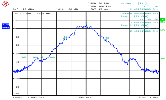
GFSK_Low 0.858MHz
