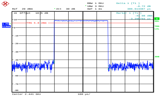
GFSK_Hopping_DH1 0.387ms
