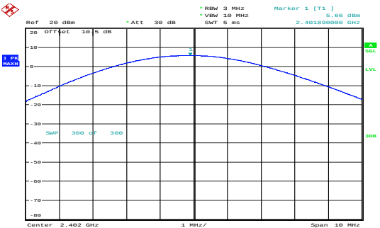
\pi/4 -DQPSK_Low 5.66dBm
