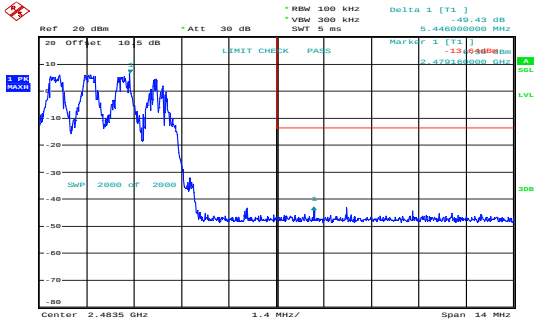
GFSK_Hopping_Upper 49.43dB
