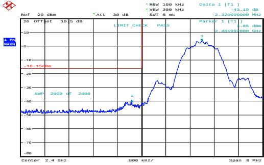
\pi/4 -DQPSK_Low 43.19dB
