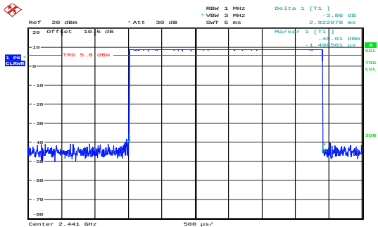
GFSK_Hopping_DH5 2.922ms
