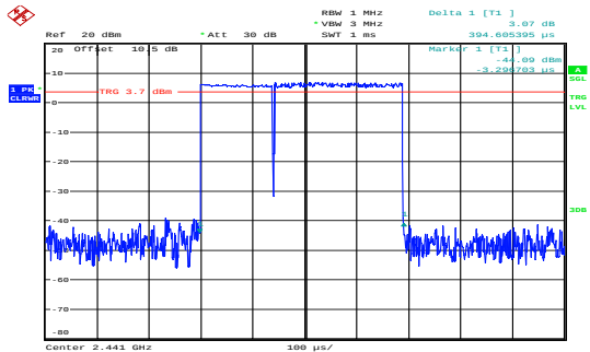
\pi/4 -DQPSK_Hopping_2DH1 0.395ms
