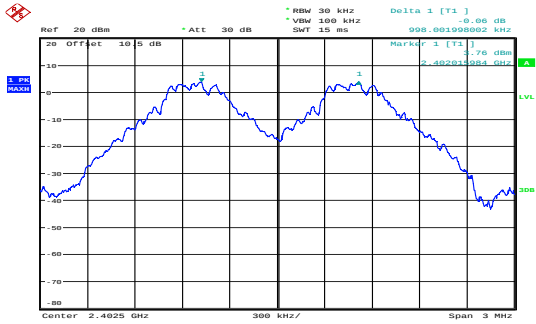
GFSK_Low 0.998MHz
