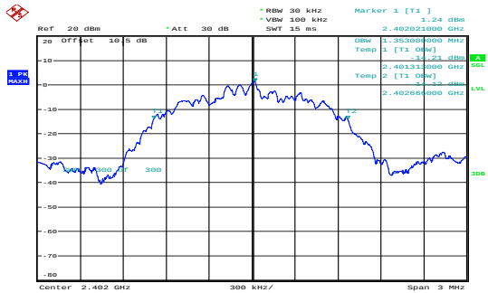
\pi/4 -DQPSK_Low 1.353MHz
