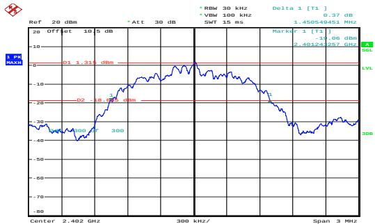
\pi/4 -DQPSK_Low 1.451MHz
