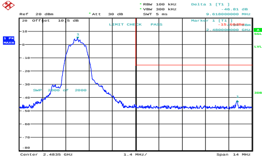
\pi/4 -DQPSK_High 46.81dB
