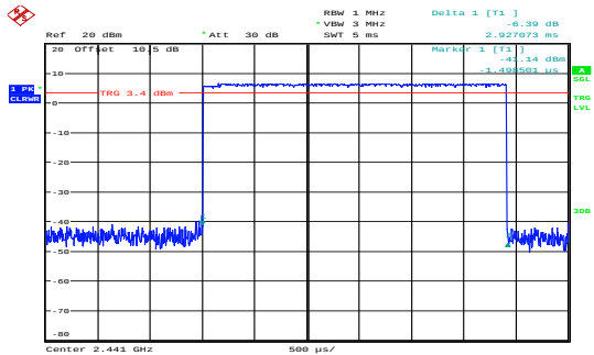
\pi/4 -DQPSK_Hopping_2DH5 2.927ms
