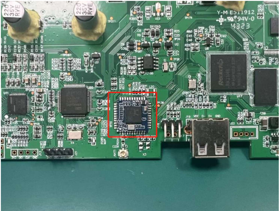
WIFI&BT Module
