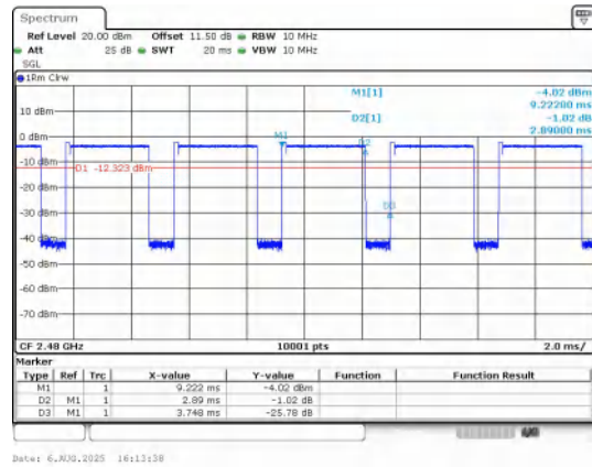
\pi/4 DQPSK(2-DH5)_Channel 78
