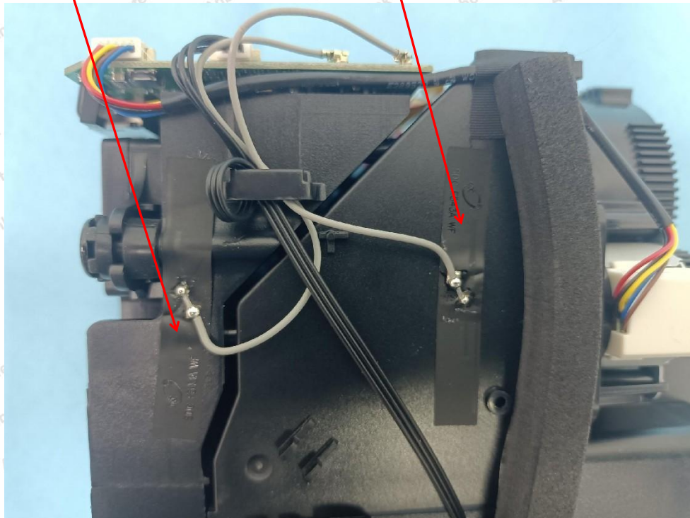
Wi-Fi ANT
