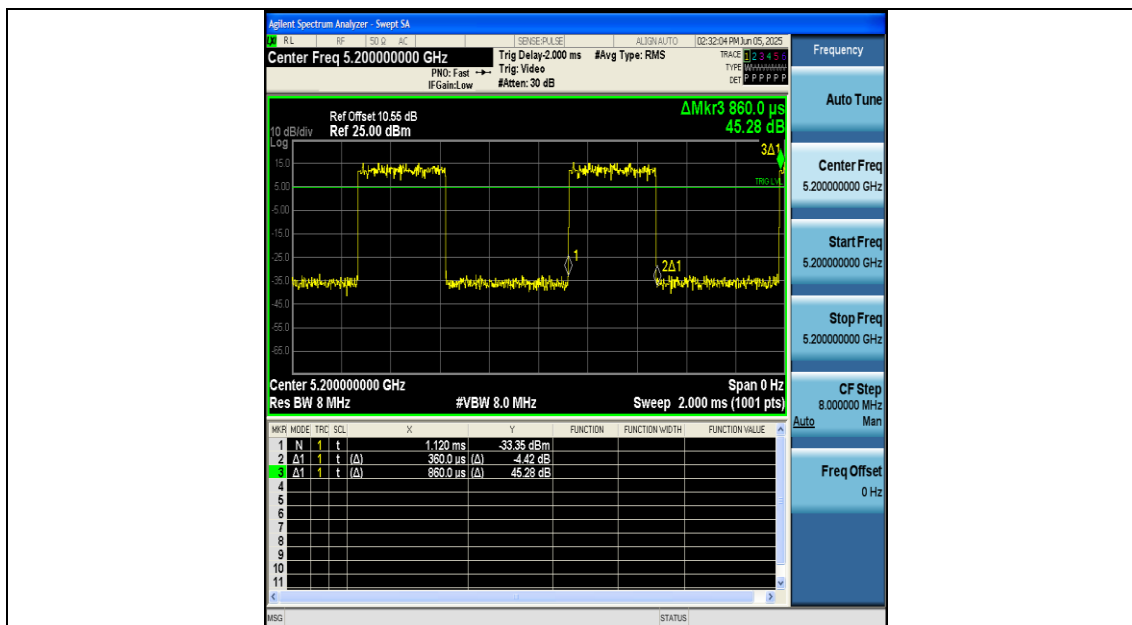
NTNV-11AC20MIMO-Ant1-5200
