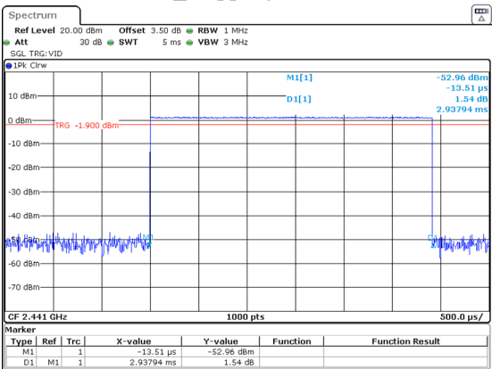
DH5_Hopping 2.938ms
