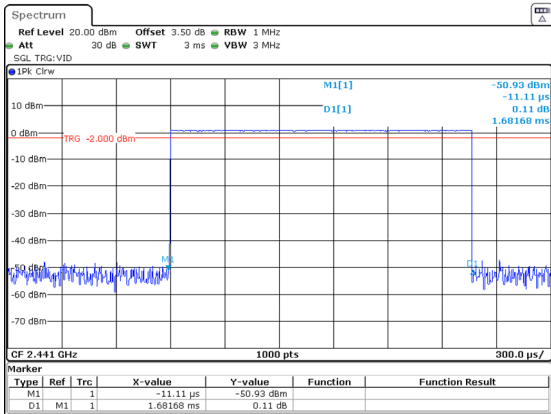
DH3_Hopping 1.682ms
