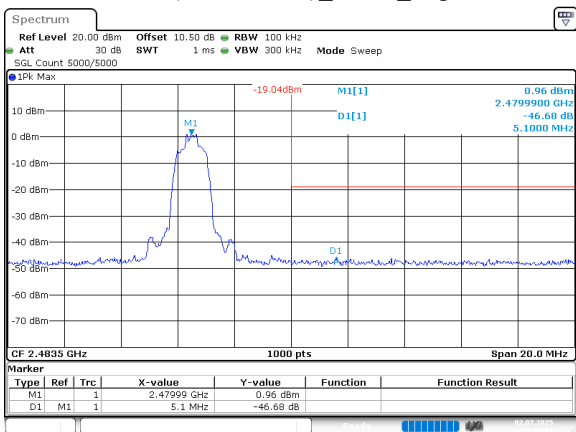
EDR( \pi/4 -DQPSK)_2DH1_High
