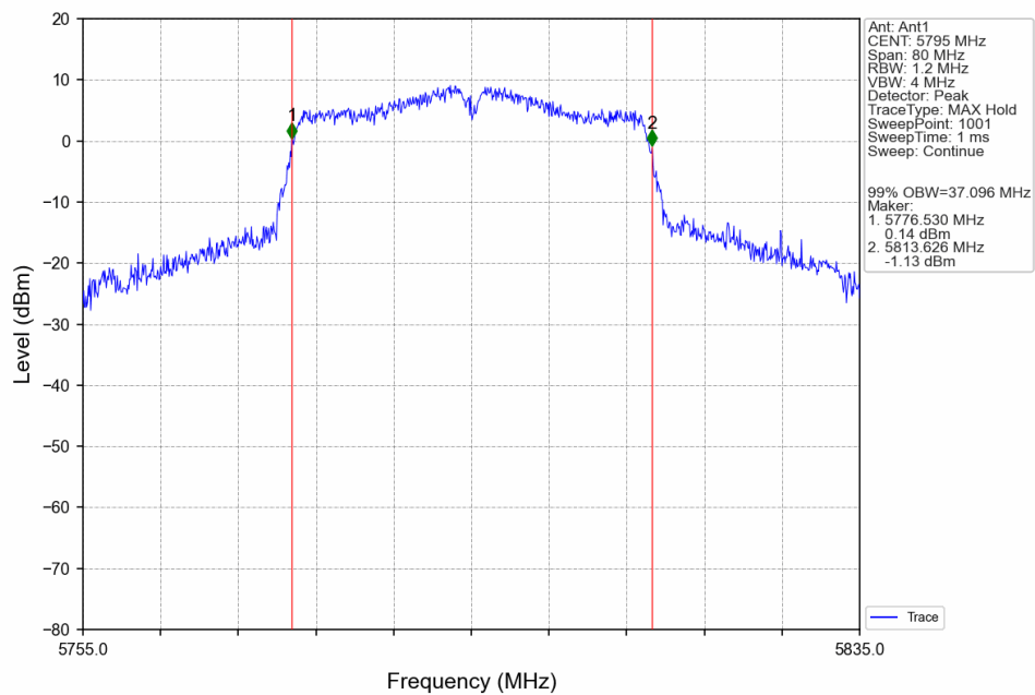
802.11ac(VHT40) HCH 5795MHz Ant1 NTV
