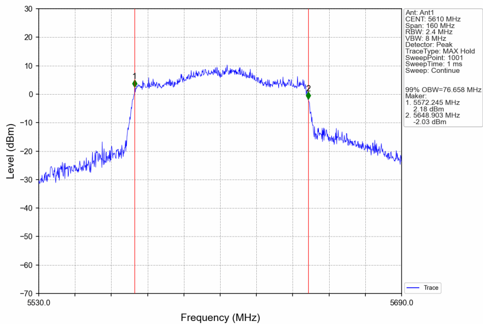
802.11ac(VHT80) HCH 5610MHz Ant1 NTV
