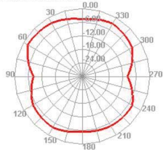
2500.000MHz H
