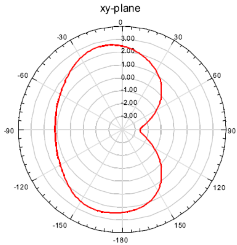
Fig 3 : Antenna Pattern
