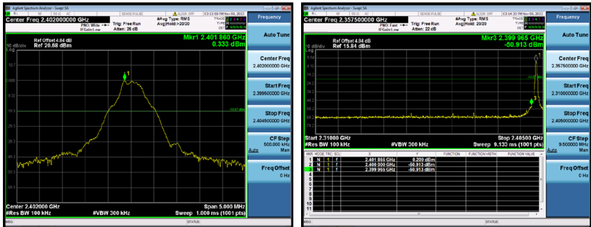
GFSK 2402MHz
