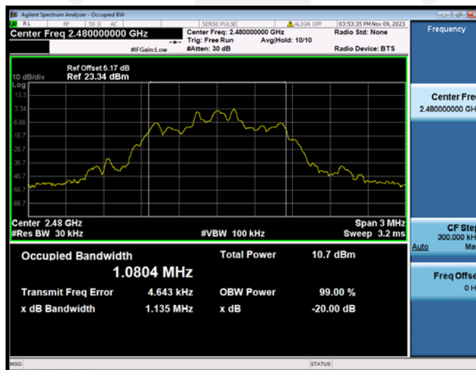
\pi/4 -DQPSK (2-DH1) 2480MHz
