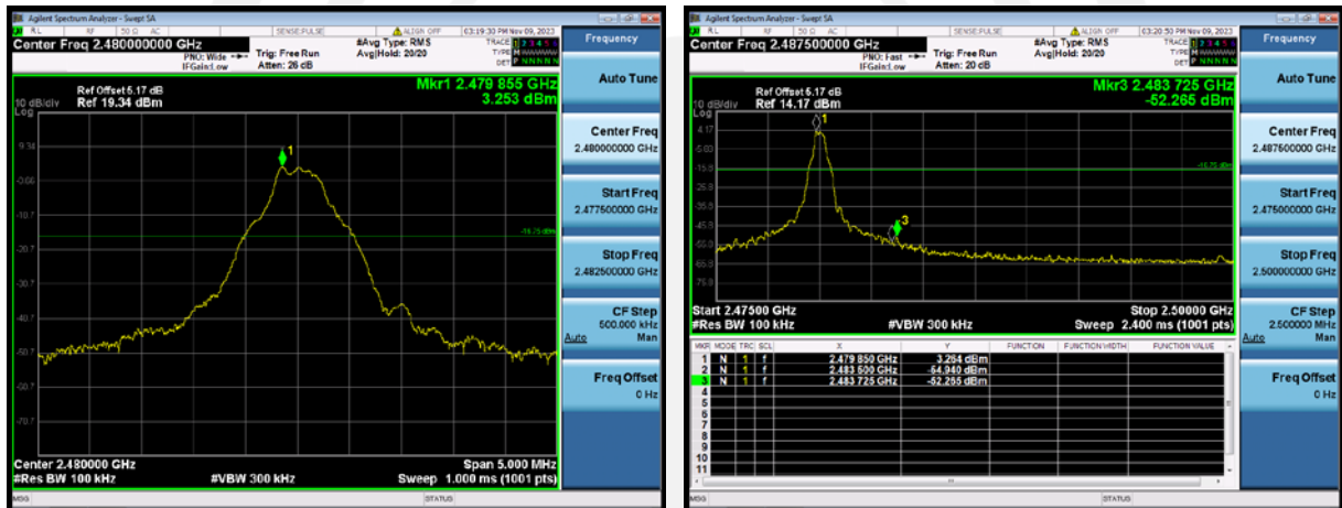
GFSK 2480MHz
