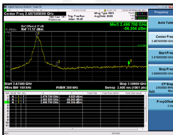
GFSK 2480MHz
