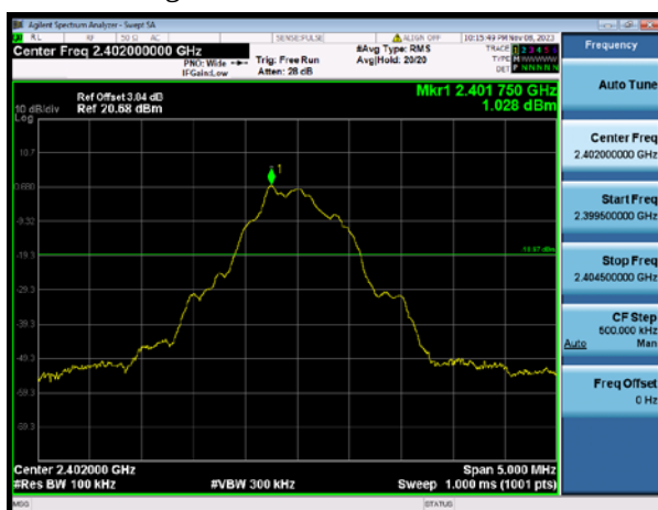
GFSK 2402MHz
