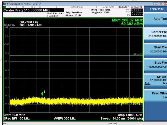
2.4G-Ant1-2402-30~1000-PASS
