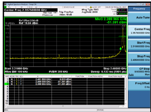
GFSK 2402MHz
