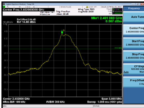
GFSK 2402MHz
