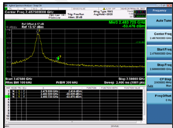
GFSK 2480MHz
