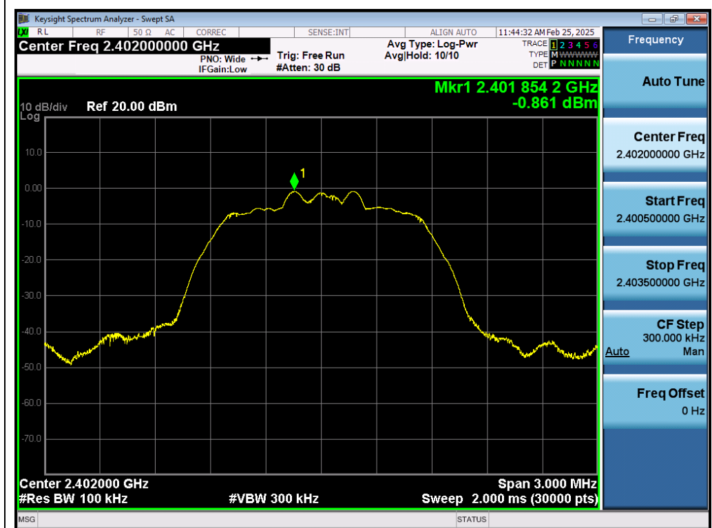
Test_Graph_EDR_ANT1_2402_2Mbps_Reference Level
