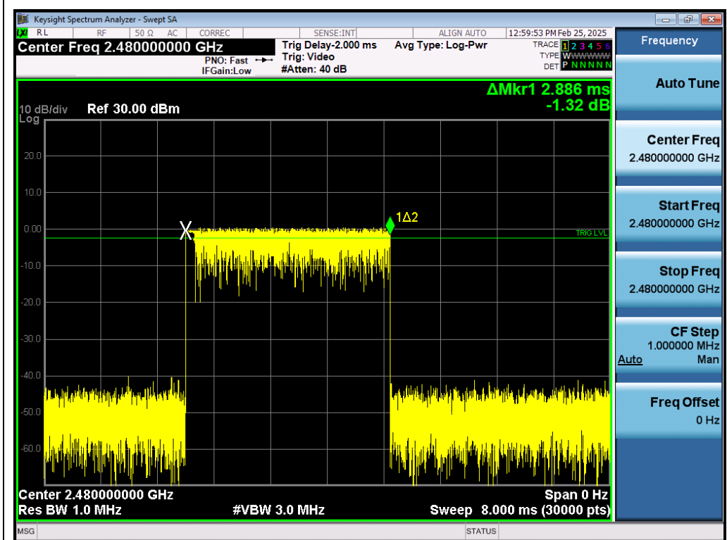
Test_Graph_EDR_HOP_ANT1_NA_3Mbps_2480_Time per Burst
