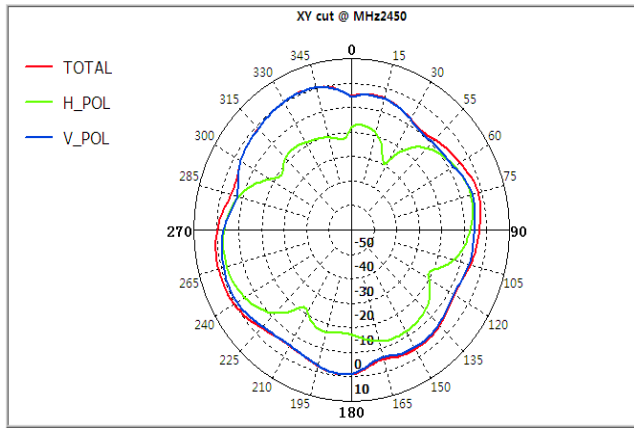
XOY-plane@2450MHz
