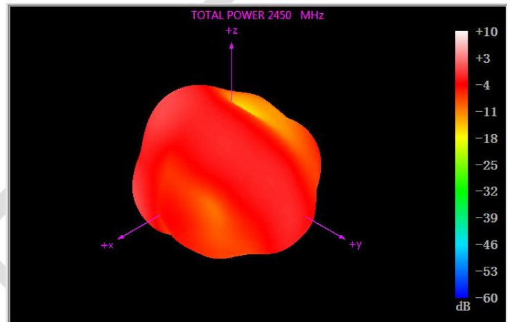
3D-plane@2450MHz
