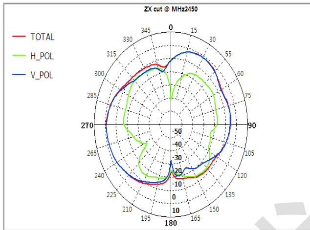
XOZ-plane@2450MHz
