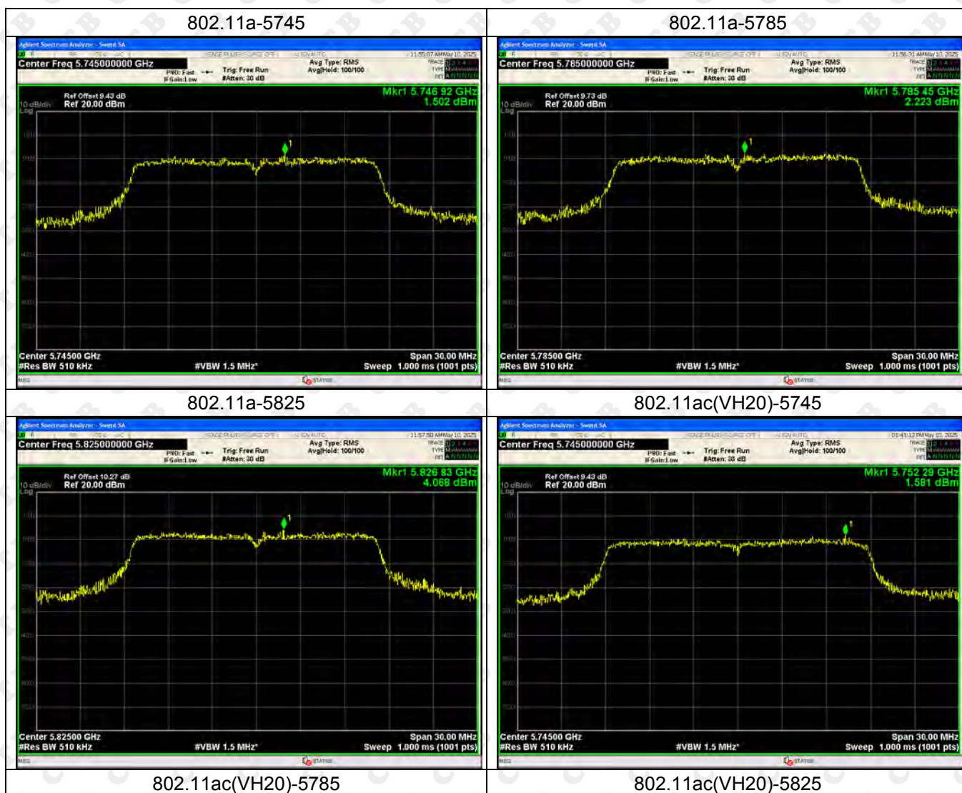
5745-5825MHz
