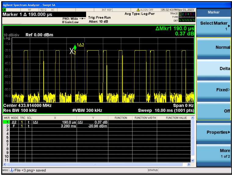
(Time per burst: 0.190ms*28pcs)
