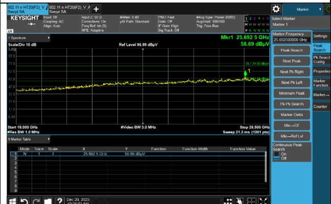
802.11 n HT20 / 2 442 MHz / (18 ~ 26.5) GHz(AV / Ver)
