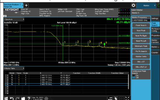
802.11 n HT20 / 2 472 MHz / Band Edge(AV / Ver)
