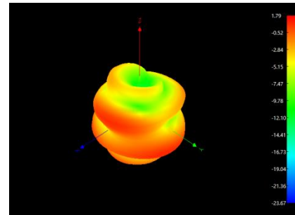
2500MHZ
