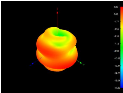
2400MHZ
