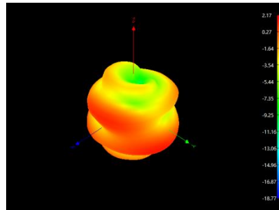
2450MHZ
