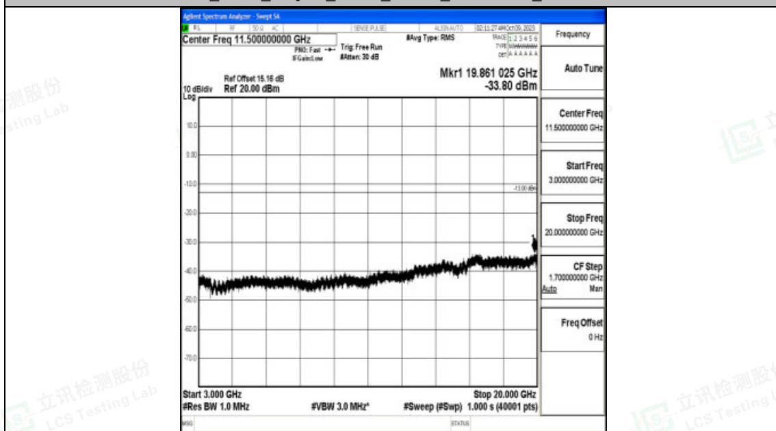
Band2 5MHz 16QAM 19175 1RB#0 3000~20000 3000~20000
