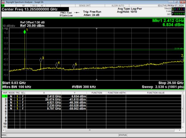
0.03GHz~26.5GHz
