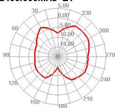
2400.000MHz E1
