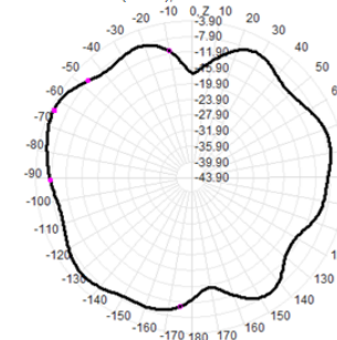
2400.0MHz Total(E2-YZ), Max=-4.73dBi
