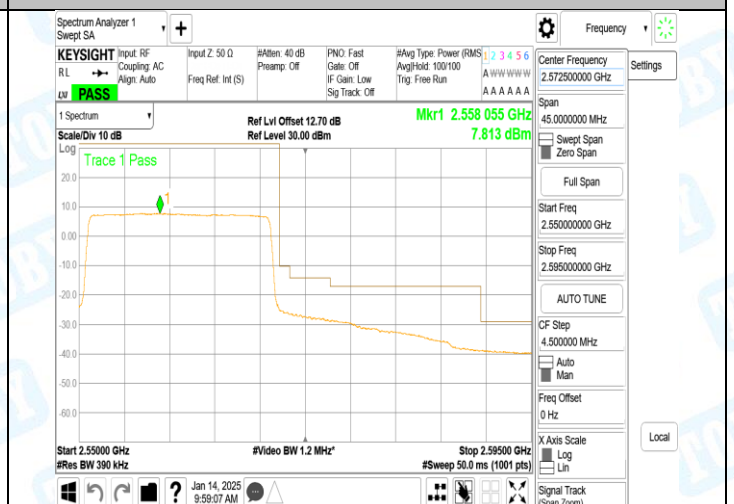
Band7_20MHz_16QAM_21350_100RB#0
