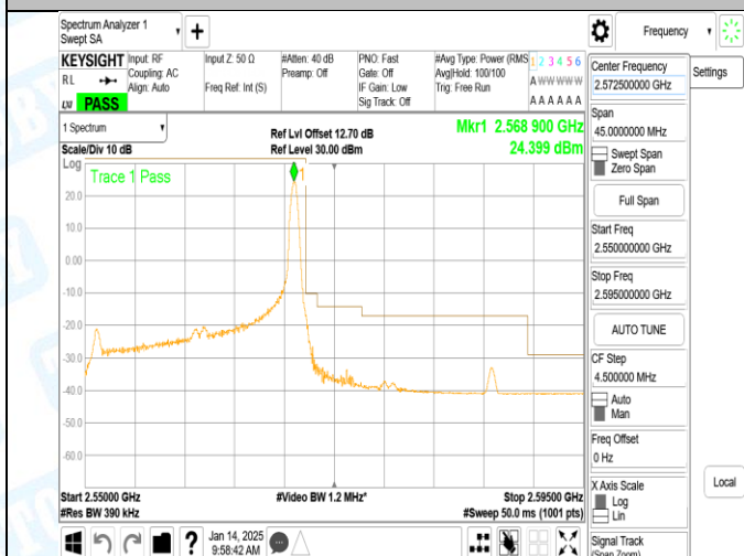
Band7_20MHz_16QAM_21350_1RB#99
