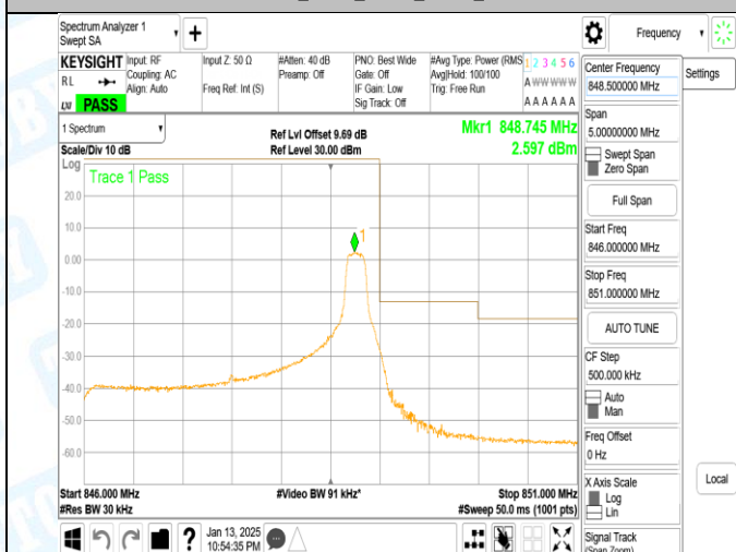
Band5_3MHz_QPSK_20635_1RB#14
