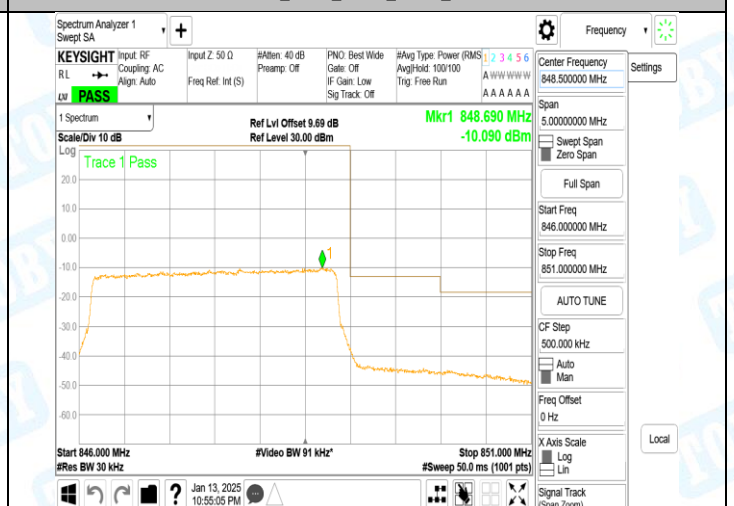
Band5_3MHz_QPSK_20635_15RB#0
