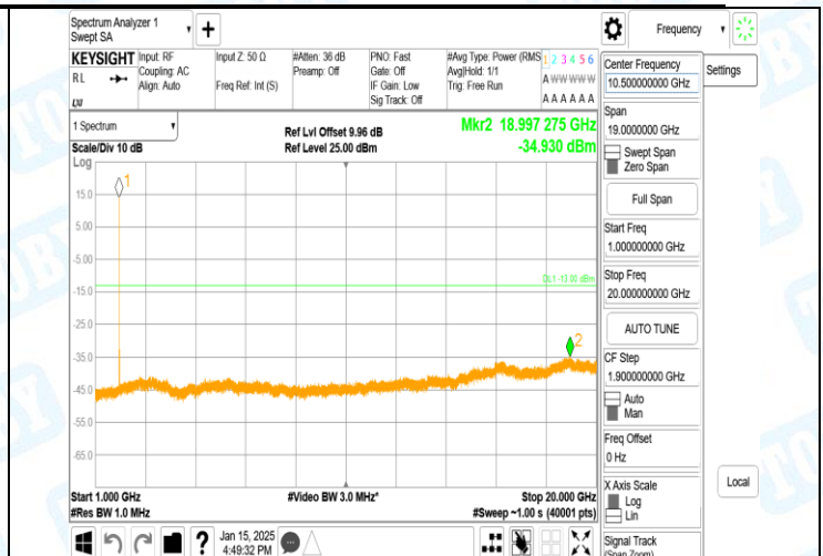
Band2-9538-1-1000~20000MHz-PASS
