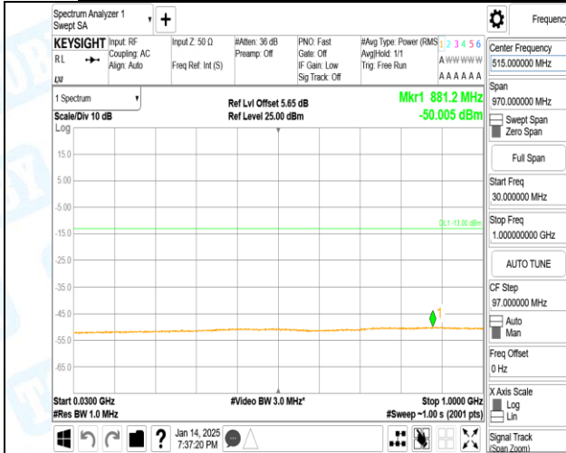
Band2-9538-3-30~1000MHz-PASS
