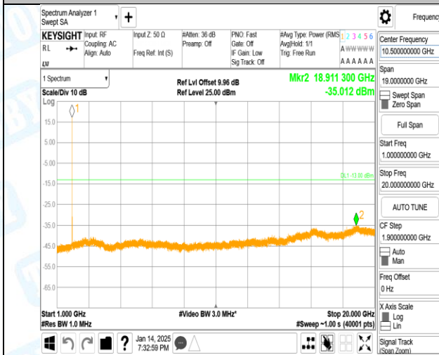
Band2-9538-1-1000~20000MHz-PASS
