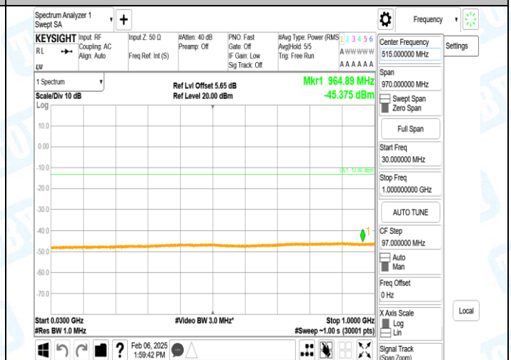
GPRS1900-661-0-30~1000MHz-PASS
