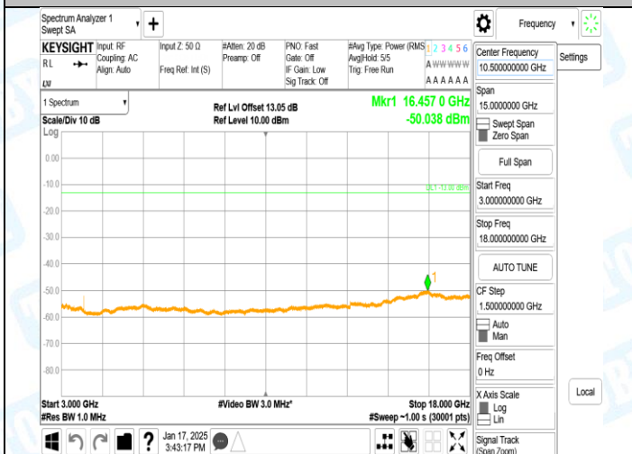
GSM1900-810-0-3000~18000MHz-PASS
