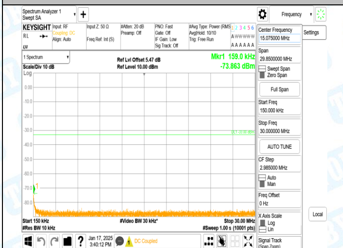
GSM1900-512-0-0.15~30MHz-PASS
