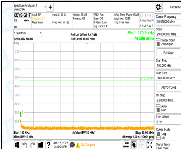
GSM1900-661-0-0.15~30MHz-PASS
