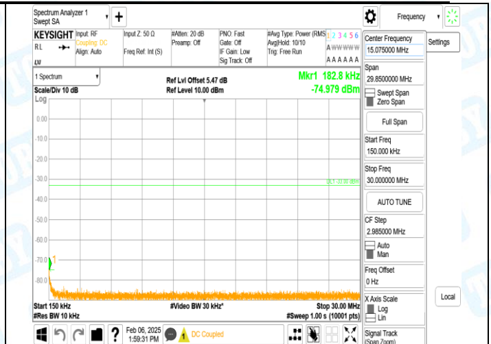
GPRS1900-661-0-0.15~30MHz-PASS
