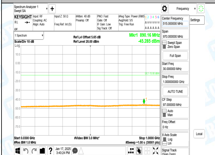
GSM1900-512-0-30~1000MHz-PASS
