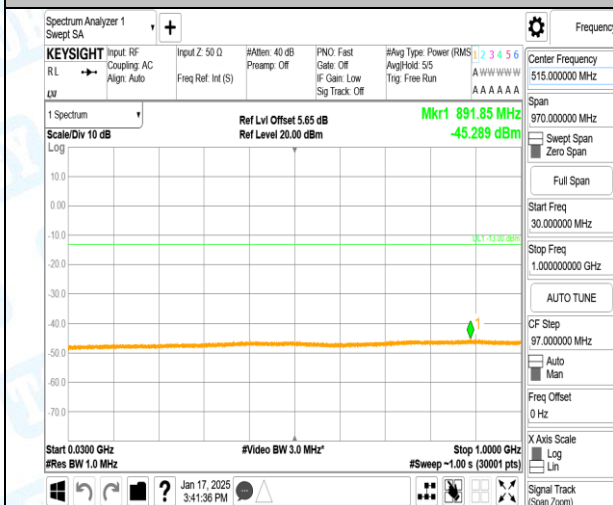
GSM1900-661-0-30~1000MHz-PASS
