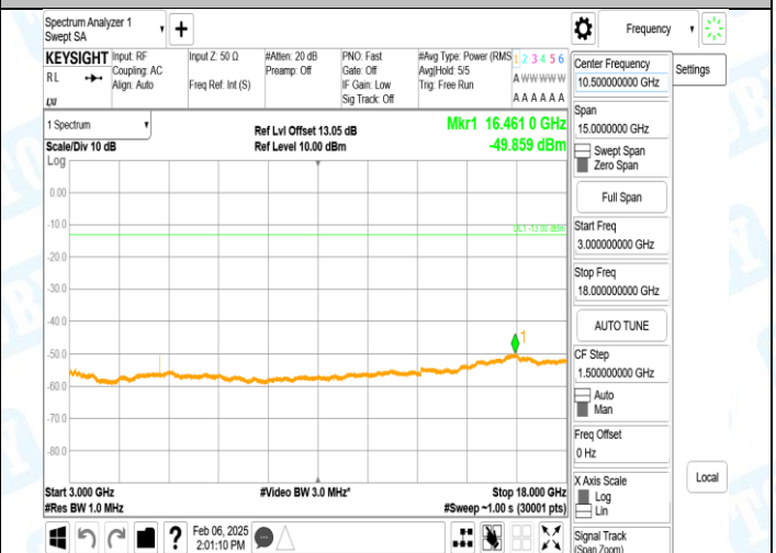
GPRS1900-810-0-3000~18000MHz-PASS
