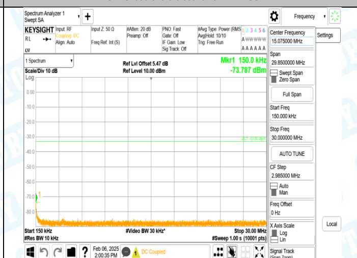
GPRS1900-810-0-0.15~30MHz-PASS
