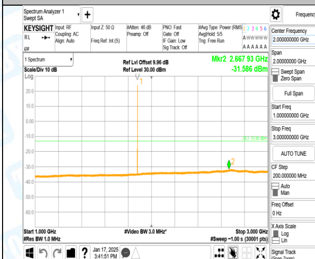
GSM1900-661-0-1000~3000MHz-PASS
