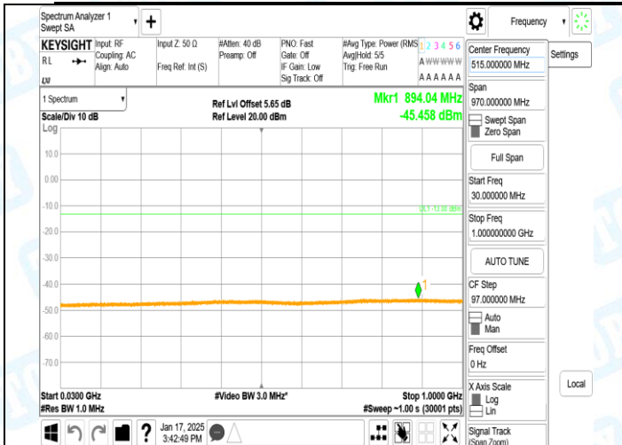
GSM1900-810-0-30~1000MHz-PASS
