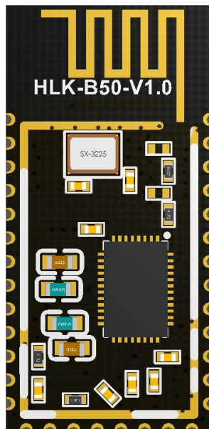
图 1: HLK-B50 板载天线位置及效果图
