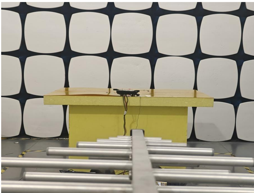
Antenna 1(IMMO) 30MHz-1GHz
