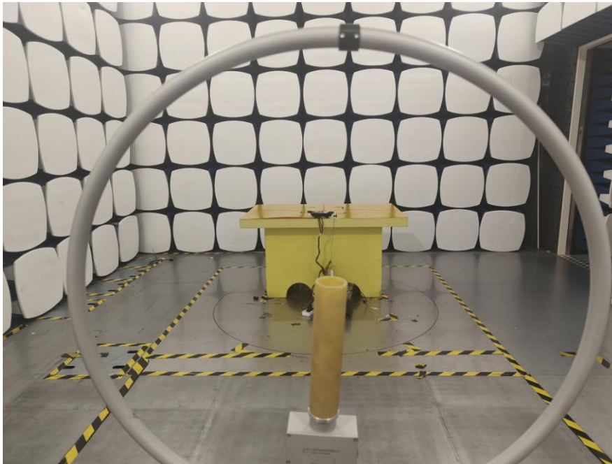
Antenna 1(IMMO) 9kHz-30MHz
