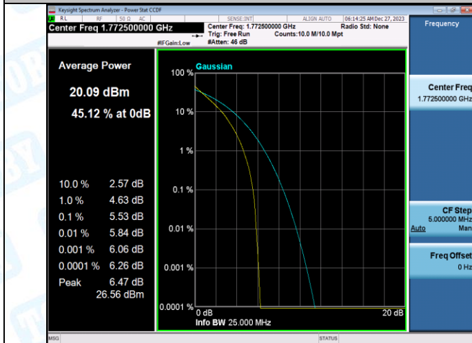
Band66-20MHz-QPSK-132072-1RB#0-PASS
