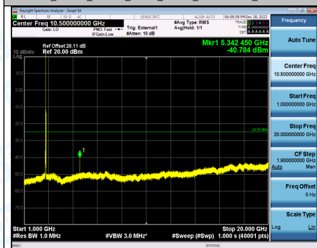
Band41 20MHz 16QAM 41490 1RB#0 1000~20000 1000~20000
