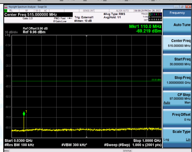
Band41 20MHz 16QAM 41490 1RB#0 20000~27000 20000~27000
