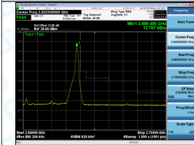
Band41_10MHz_QPSK_41540_50RB#0
