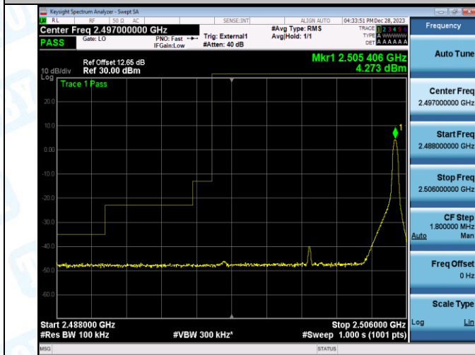
Band41_10MHz_QPSK_39700_50RB#0
