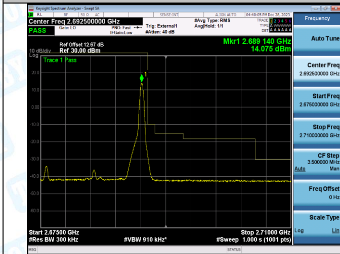
Band41_15MHz_QPSK_41515_75RB#0
