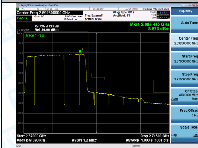
Band41_20MHz_QPSK_41490_100RB#0
