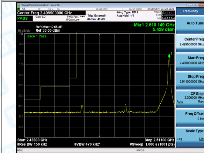
Band41_15MHz_QPSK_39725_75RB#0
