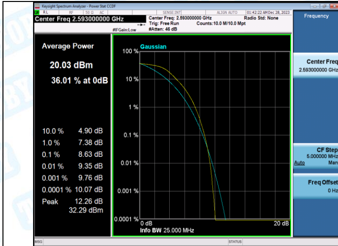
Band41-20MHz-QPSK-41490-1RB#0-PASS
