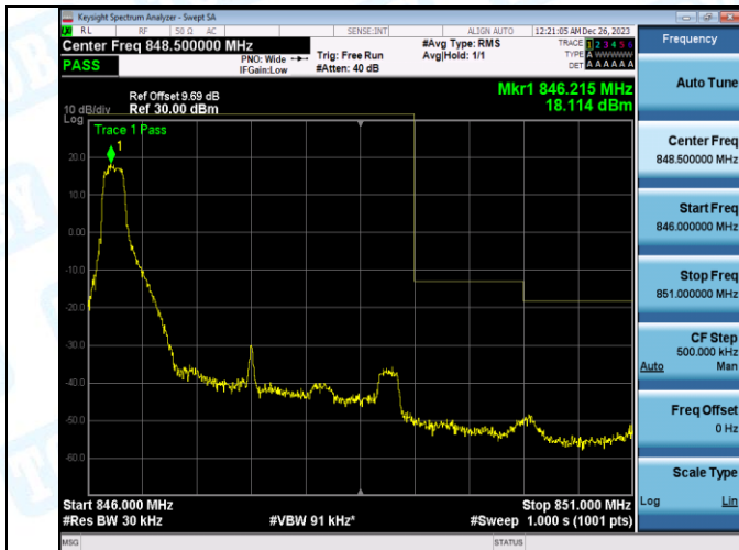
Band5_3MHz_QPSK_20635_1RB#14
