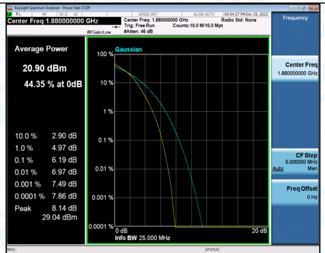
Band2-20MHz-16QAM-19100-1RB#0-PASS
