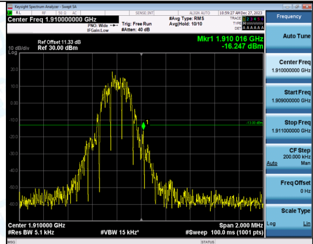
GPRS1900-810-0-PASS
