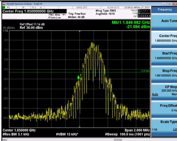
GPRS1900-512-0-PASS
