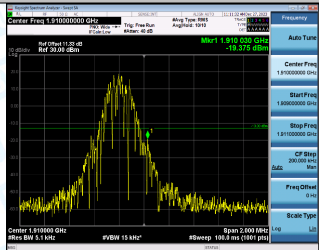
EGPRS1900-810-2-PASS
