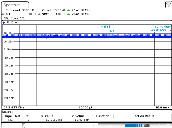
802.11g_2437MHz
