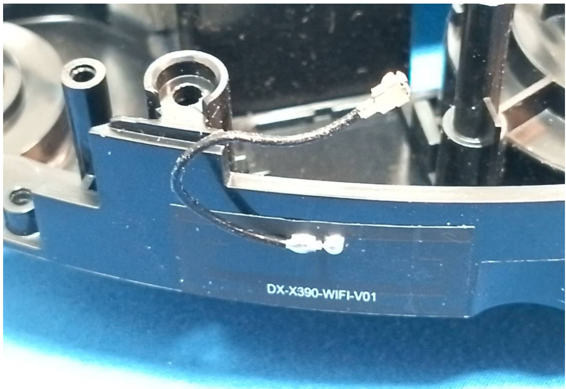
Bluetooth&Wifi Antenna
